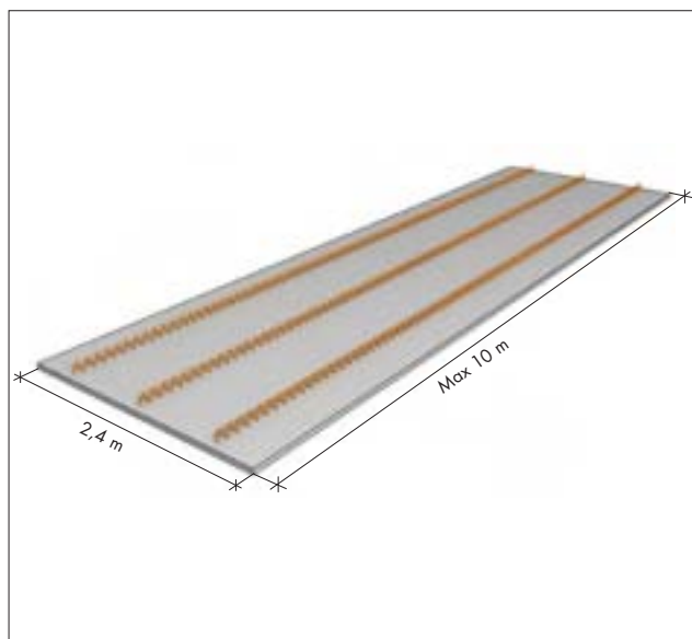
Plan plattbärlag
