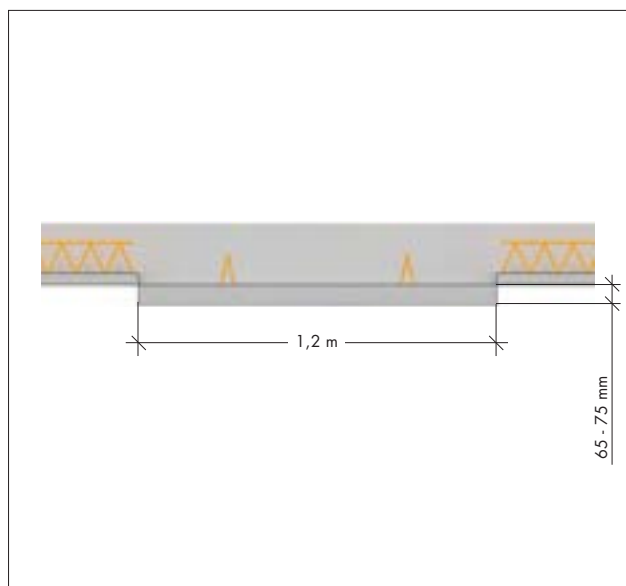
Sektion plattbärlagsbalk
