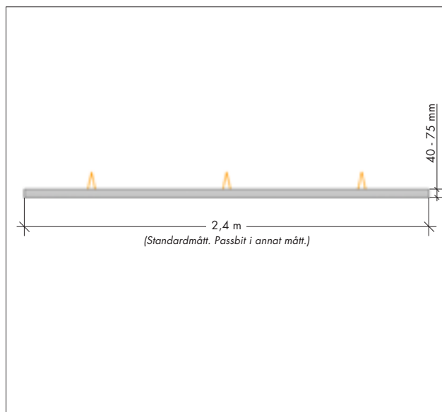
Sektion plattbärlag
