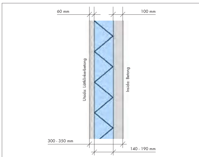
Sektion LK Putsvägg
