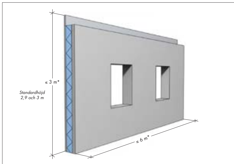
Väggelevation normalelement
