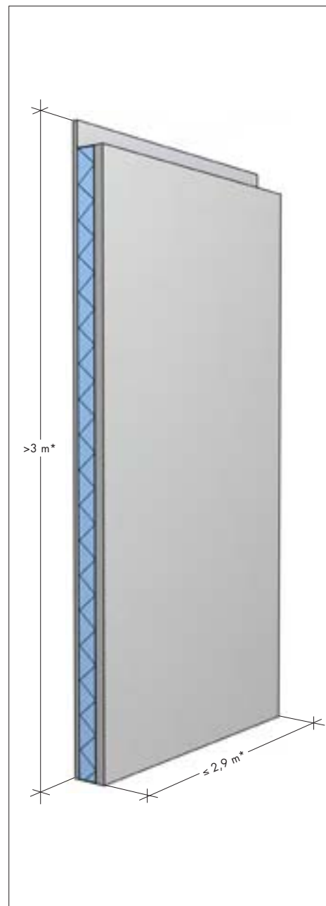
Väggelevation vändelement
