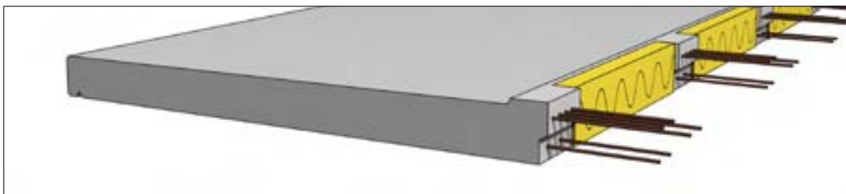
Inspänd med intermittent isolering (utstickande armering)
